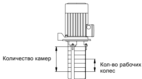
Рис. 28 Насос MTH
