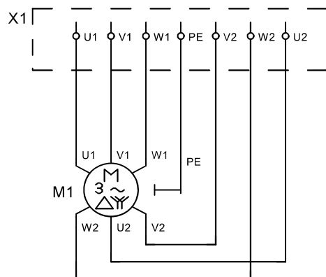
Подключение двигателя мешалки
